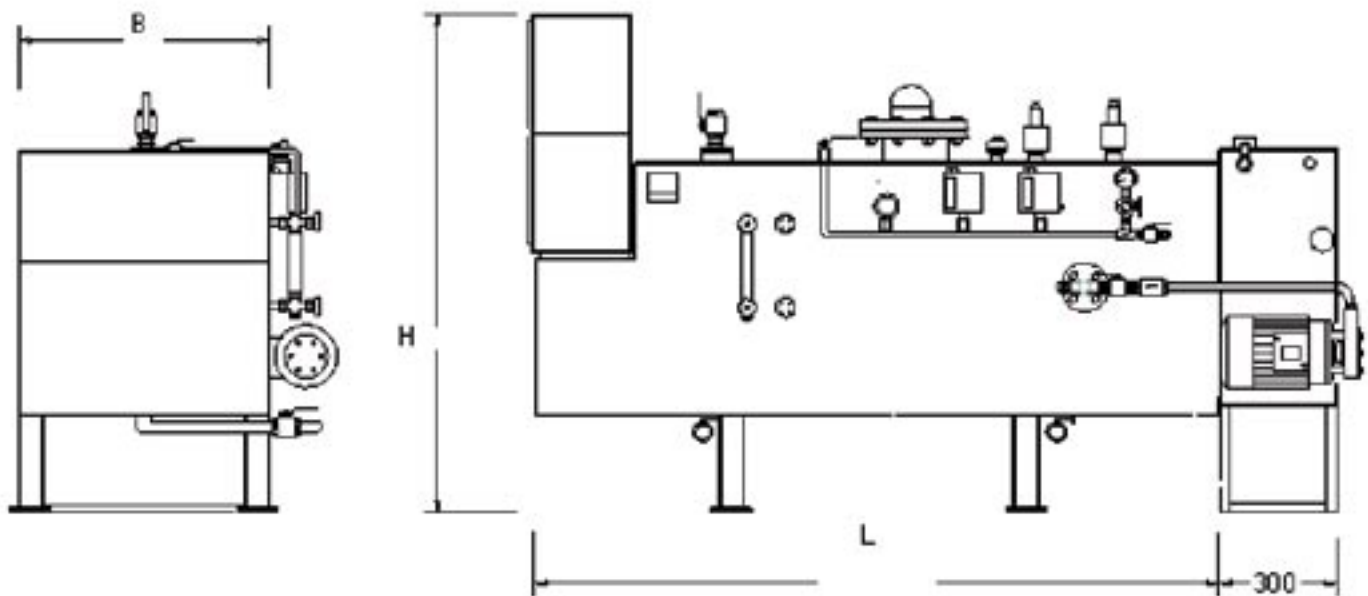
Utförande med matarvattentank och pump
